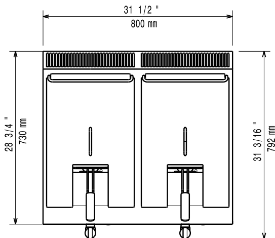
Felülnézet
